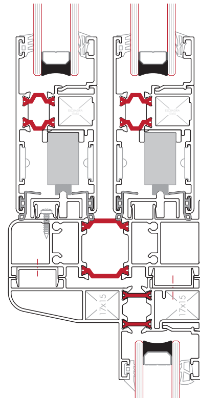
CERCO INFERIOR - FIJO ESCALA 1:2
