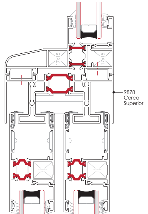
CERCO SUPERIOR - FIJO ESCALA 1:2
