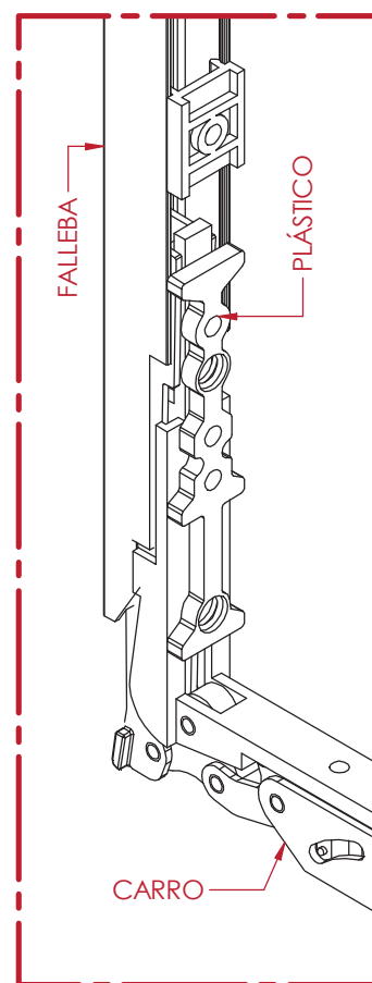
DETALLE J
